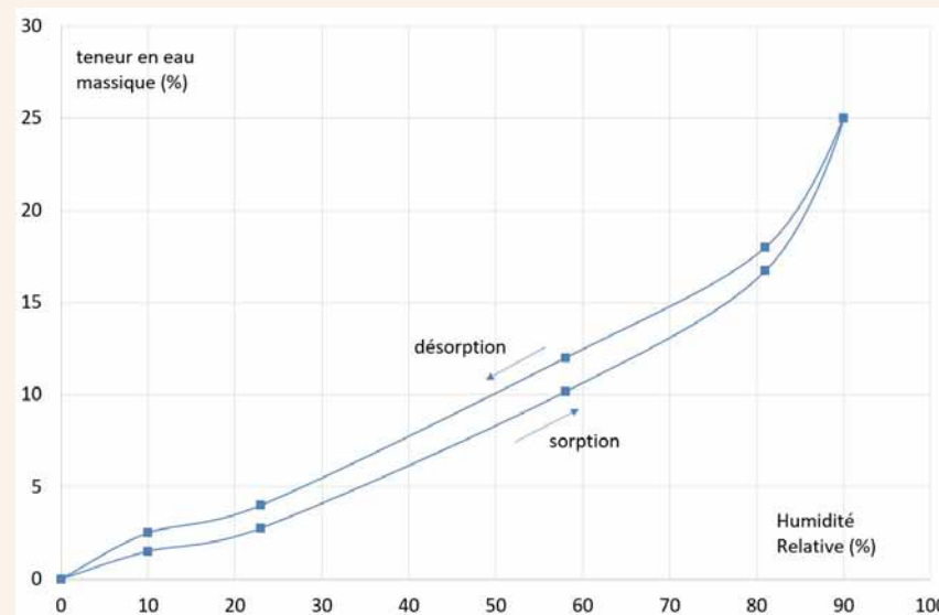
Isothermes de sorption et désorption
